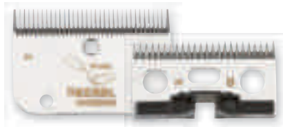
18916 Schermesser-Set R22 hautnaher Schnitt ca. 0,5 mm
